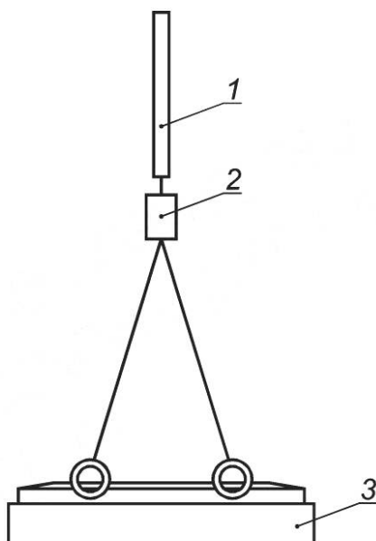
Рисунок Ж.3 — Испытательная система
